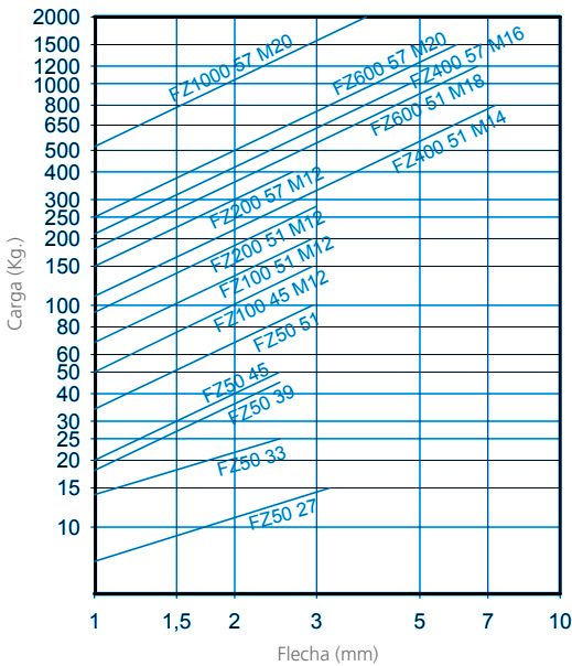
CURVAS DE CARGA FLECHA AMC MECANOCAUCHO® FZ+SYLOMER®
